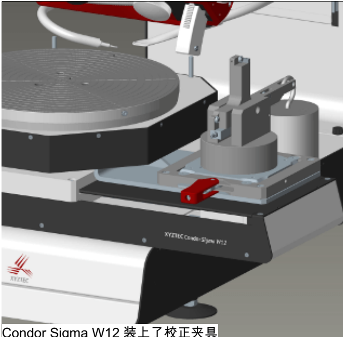
Condor Sigma W12 装上了校正夹具
