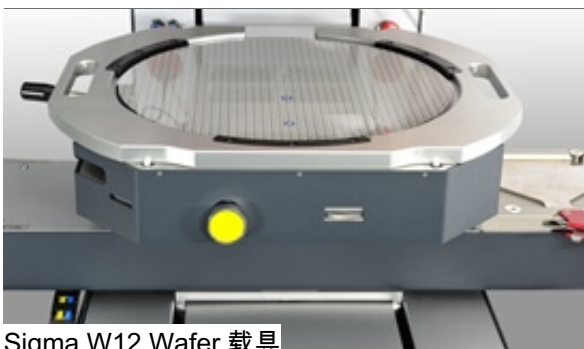
Sigma W12 Wafer 载具
