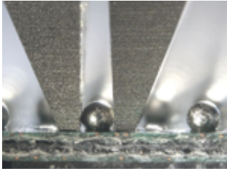
CBP Tweezer 夹子准备关上
