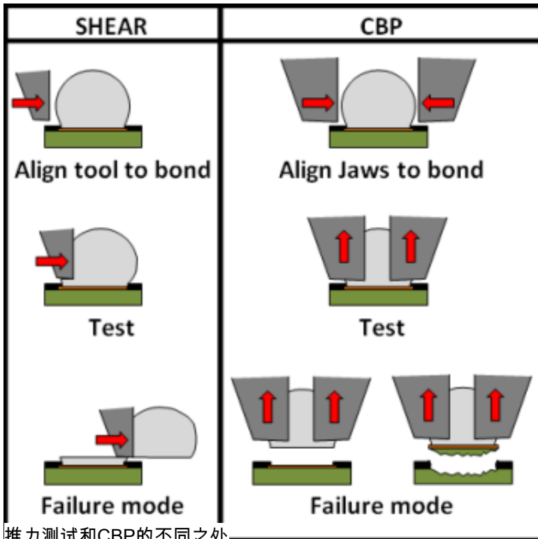
推力测试和CBP的不同之处
