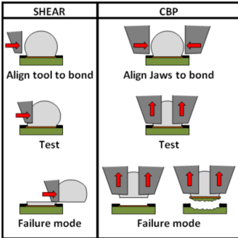
Shear 테스트와 CBP 테스트의 차이
