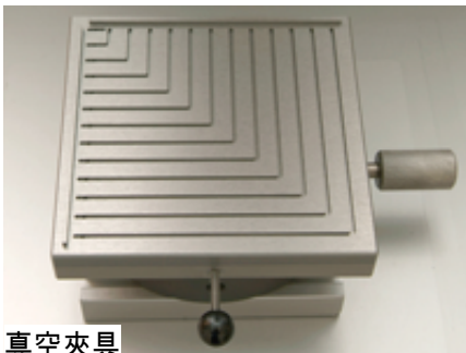
真空夾具
